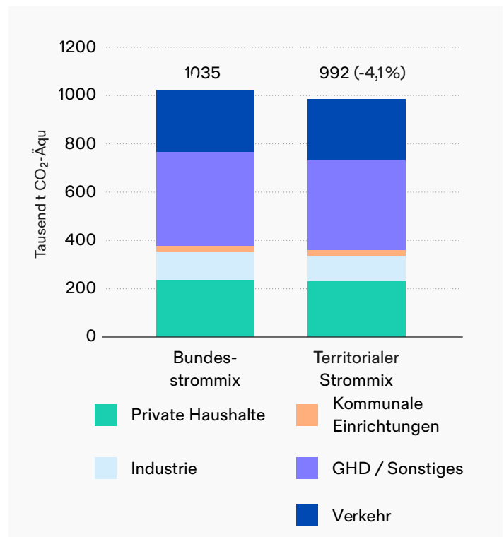
Abbildung 4: Beitrag des territorialen Strommix zur Basisbilanz mit Bundesstrommix (Quelle: eigene Darstellung)
